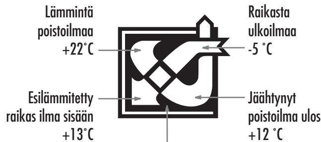
LÄMMÖN TALTEENOTTOLAITE
